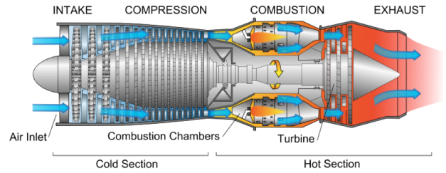
İtki Sistemleri
