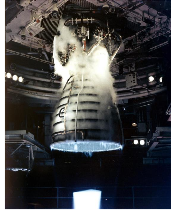
Uzay mekiği ana motorunun test ateşlemesi (Kaynak: Wikimedia Commons)
