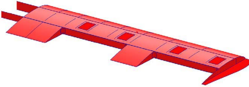
Şekil 5. Kanat taşıyıcı kısmının geometrik modelinin dış görünümü
